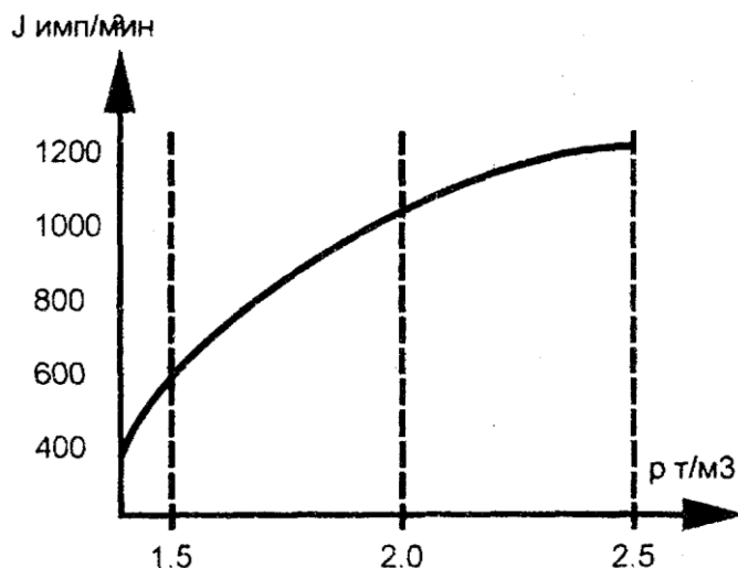
Рис. 6. Тарировочная зависимость.
